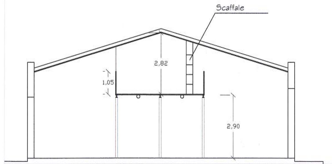
SEZIONE A-A'
